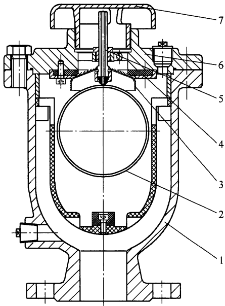
图 1 微量进排气阀
