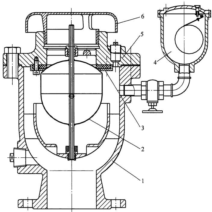
图 2 快速进排气阀
