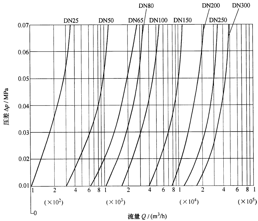
图 A.1 进排气阀排气量曲线图
